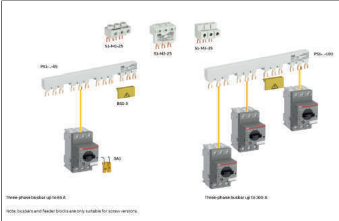
Accessories for MS116 MS132 และ MO132
